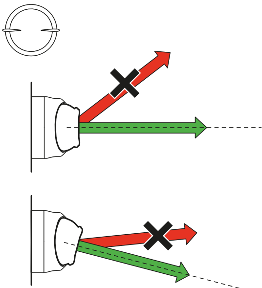
Sensore con orientamento orizzontale (volumetrico).
