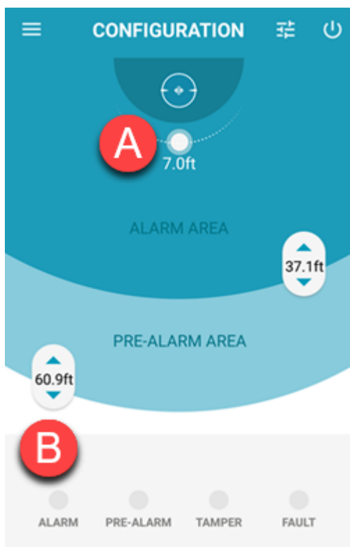
Calibrazione errata. Valore di calibrazione troppo alto.
