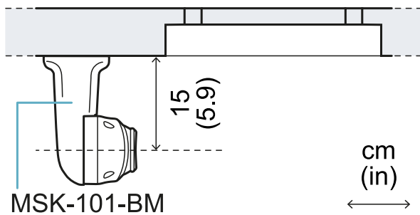
Esempio installazione con adattatore MSK-101-BM.
